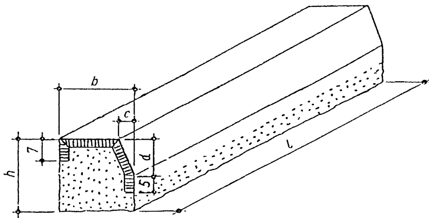
Rys. 3. Krawężnik mostowy rodzaju A
