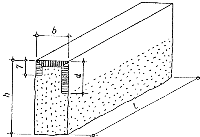
Rys. 2. odmiany UP, Tabela 2. krawężników
