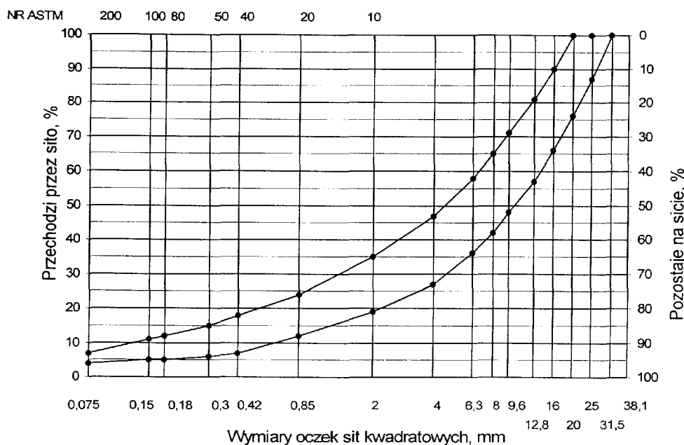
Rys. 7. Krzywe graniczne uziarnienia mieszanki mineralnej BA od 0 do 25 mm podbudowy nawierzchni drogi o obciążeniu ruchem dla KR 3.
