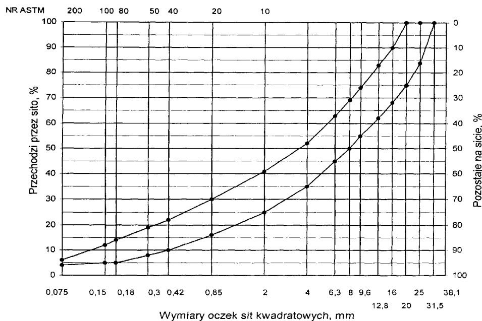
Rys. 12. Krzywe graniczne uziarnienia mieszanki mineralnej BA od 0 do 20 mm do warstwy wiążącej, wyrównawczej nawierzchni drogi o obciążeniu ruchem KR3.
